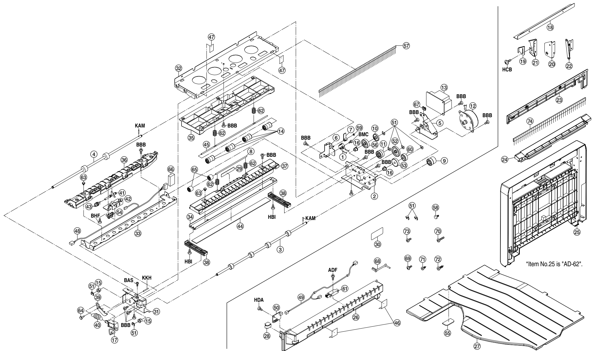
FIG. 1 DUPLEX UNIT
